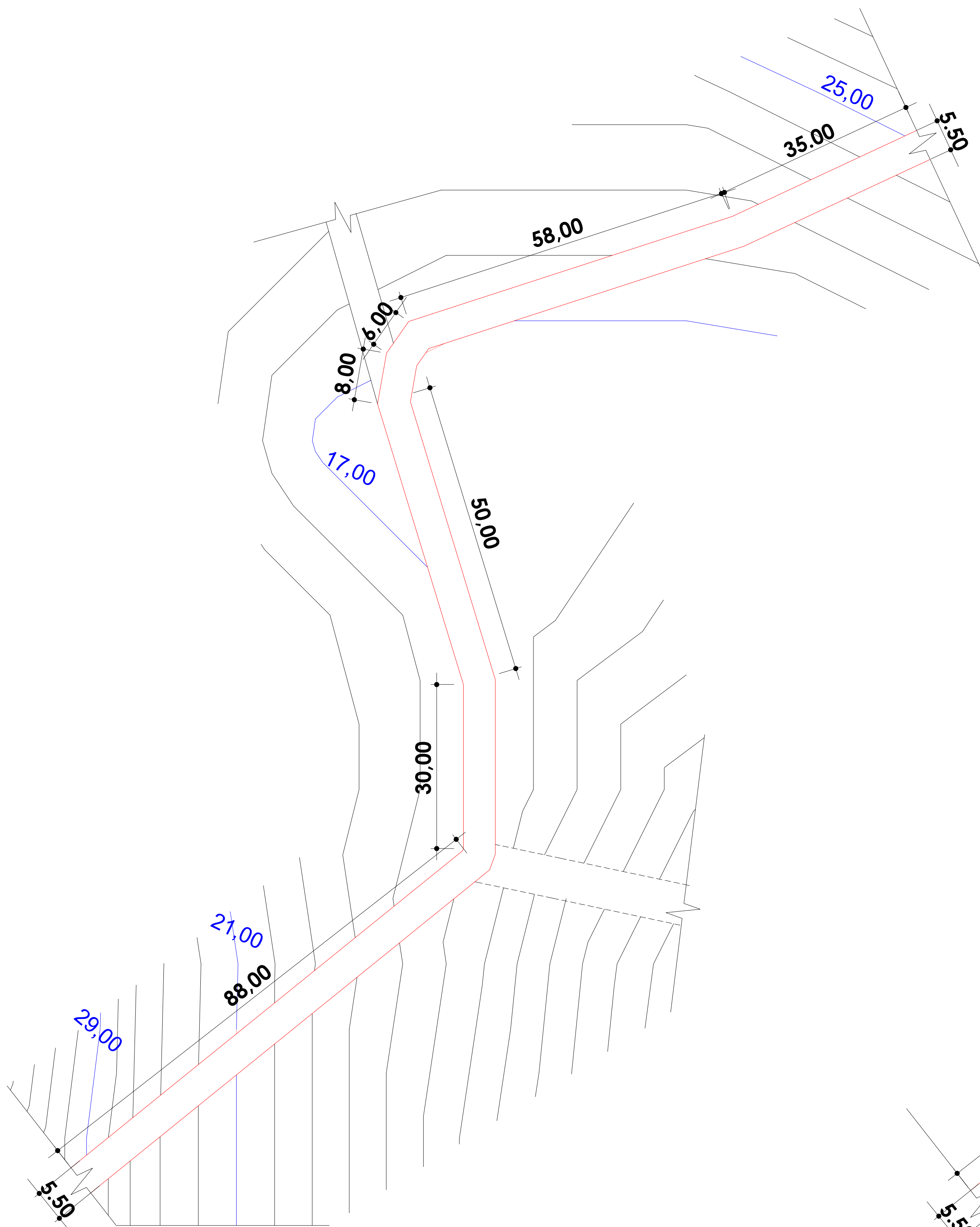
02 LEVANTAMENTO PLANIALTIMÉTRICO ESCALA: 1/700
