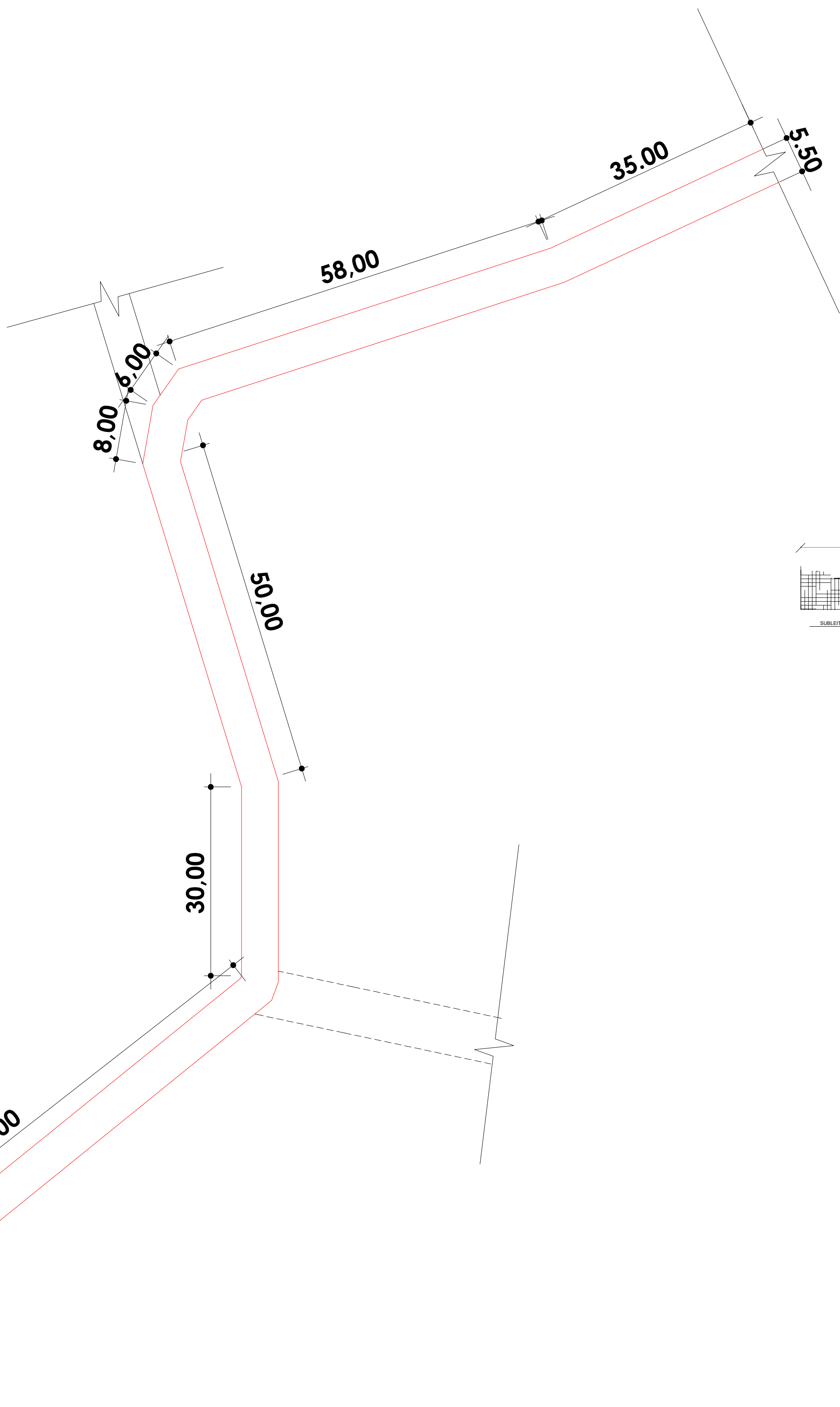
01 PLANTA LOCALIZAÇÃO
